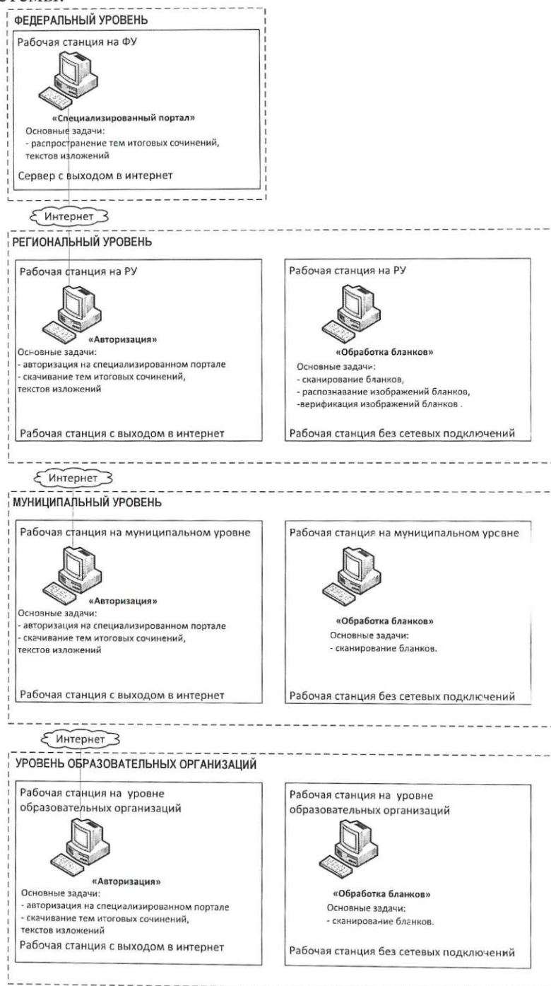
Рисунок 1 – Архитектура и состав ПО
